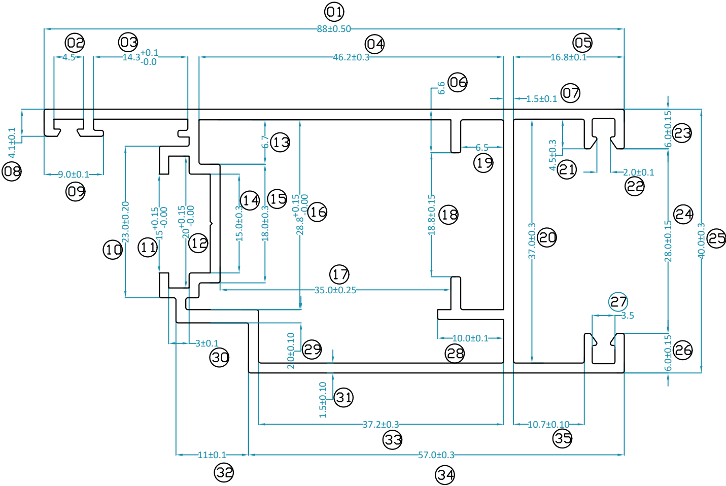
SCALE-3:1
