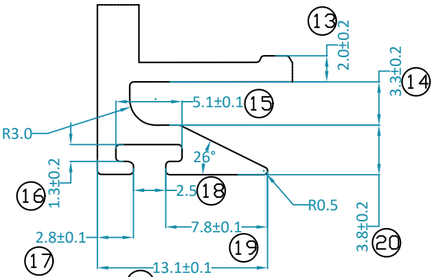
SECTION A, SCALE-3:1
