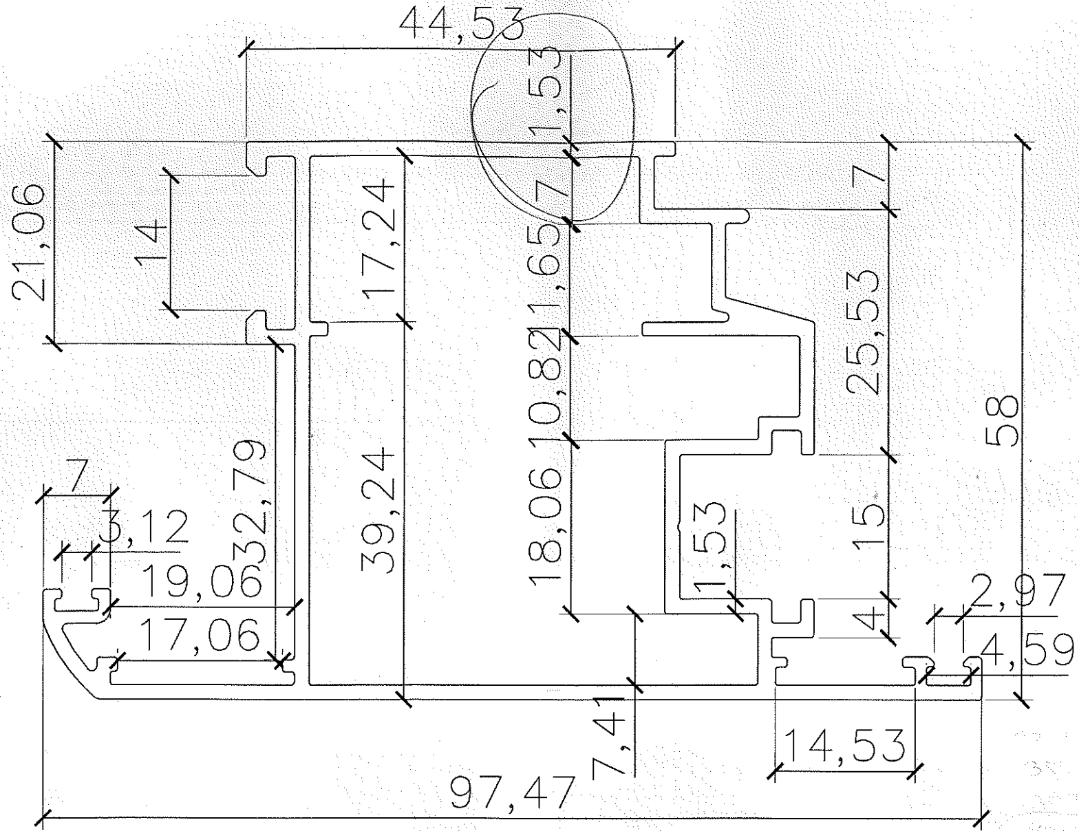
Casement Door Shutter Frame
