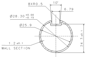
Section view A-A Scale: 2:1
