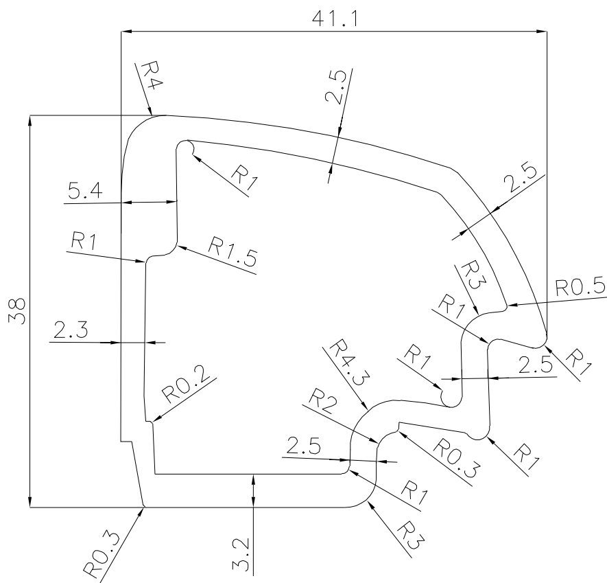
SECT : A-A (2:1)
