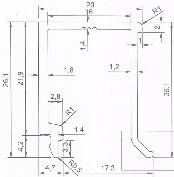
SCALE-2:1
