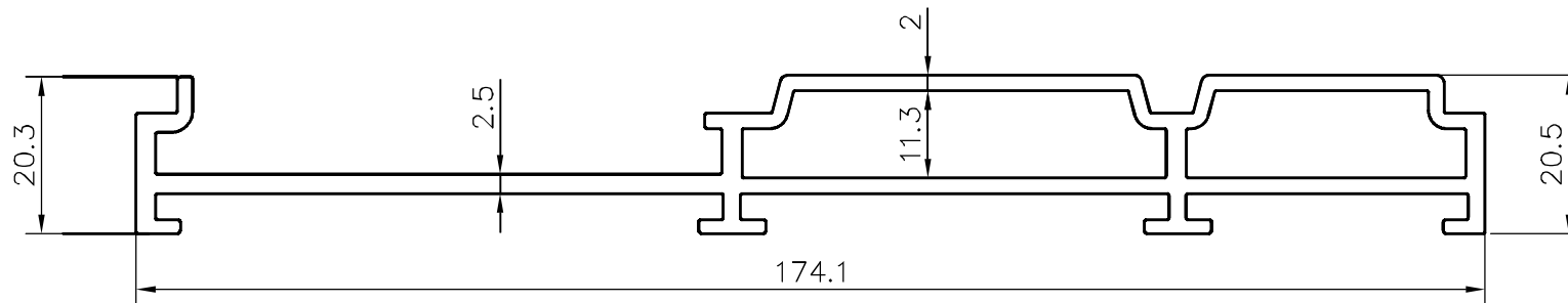
84703 3TRACK FRAME BOTTOM CLIP
