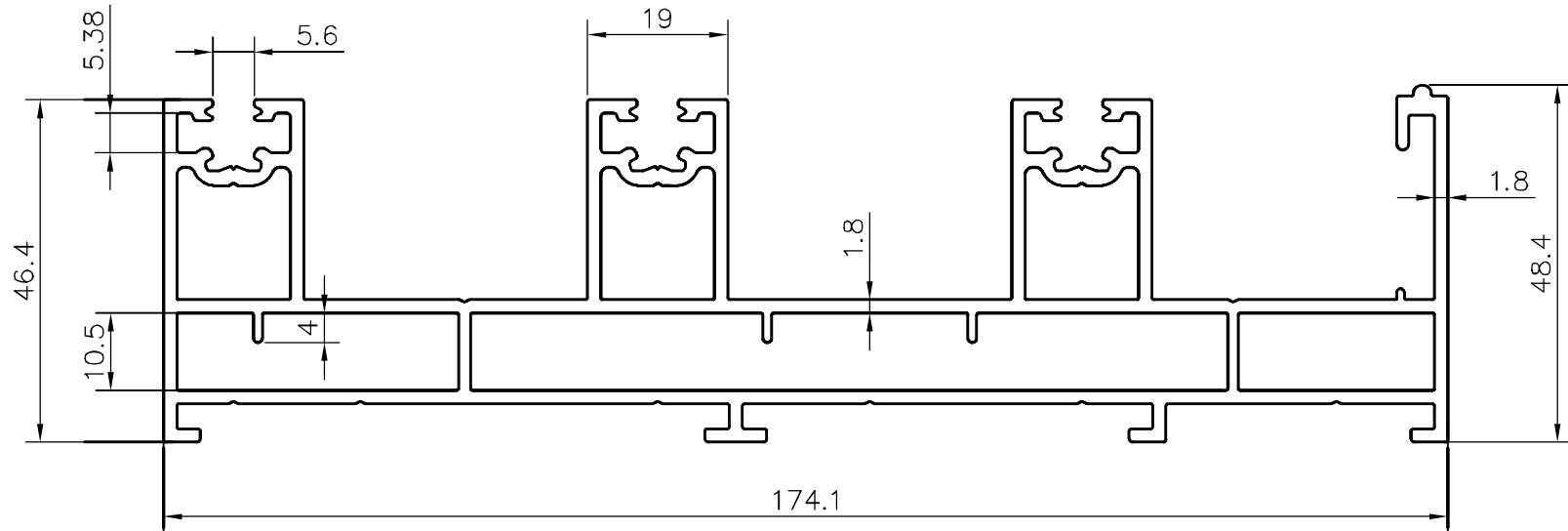
84121 3TRACK SLIDING FRAME
