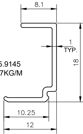
SCALE 2:1
