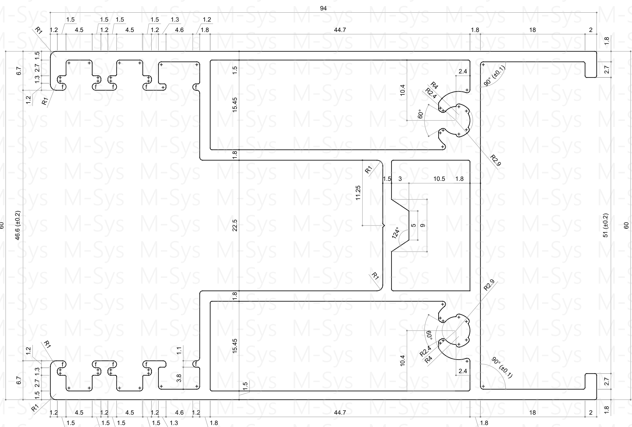
Scale 1:1
