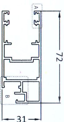
SCALE-1:1
