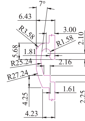
DETAILS 'A' SCALE 2:1
