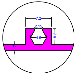
Section-A
