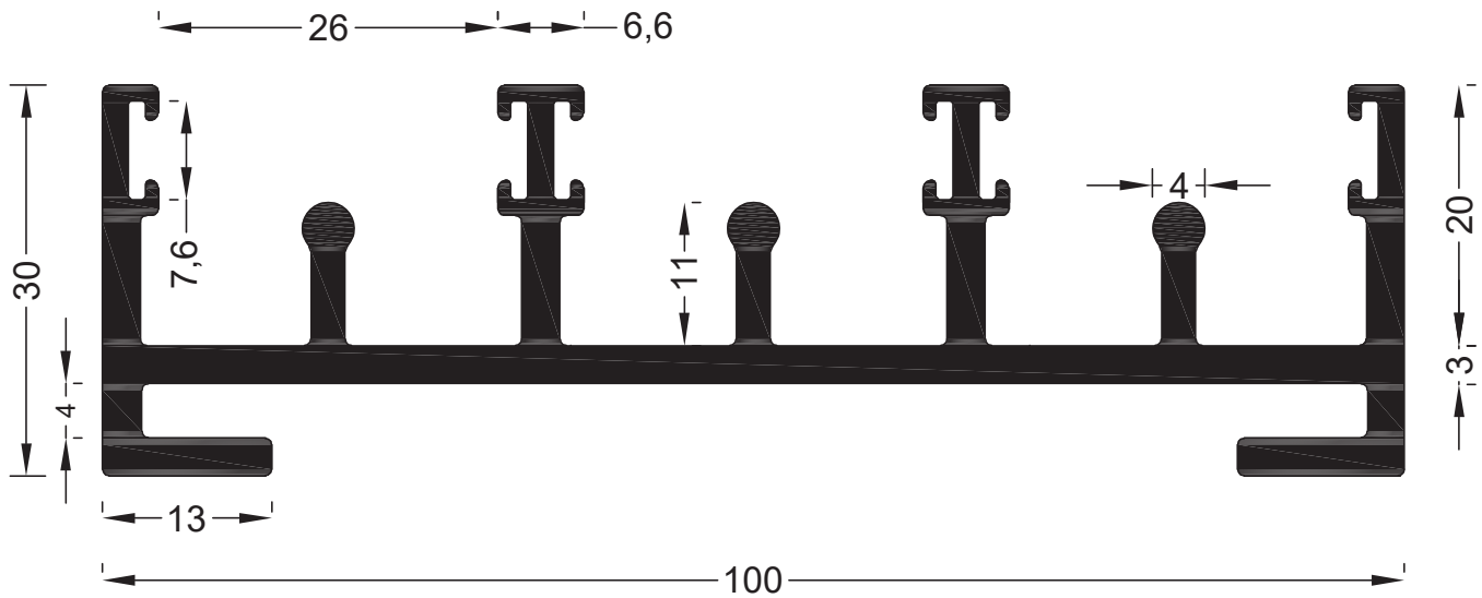
3Track Bottom 2 Kg/M approx
