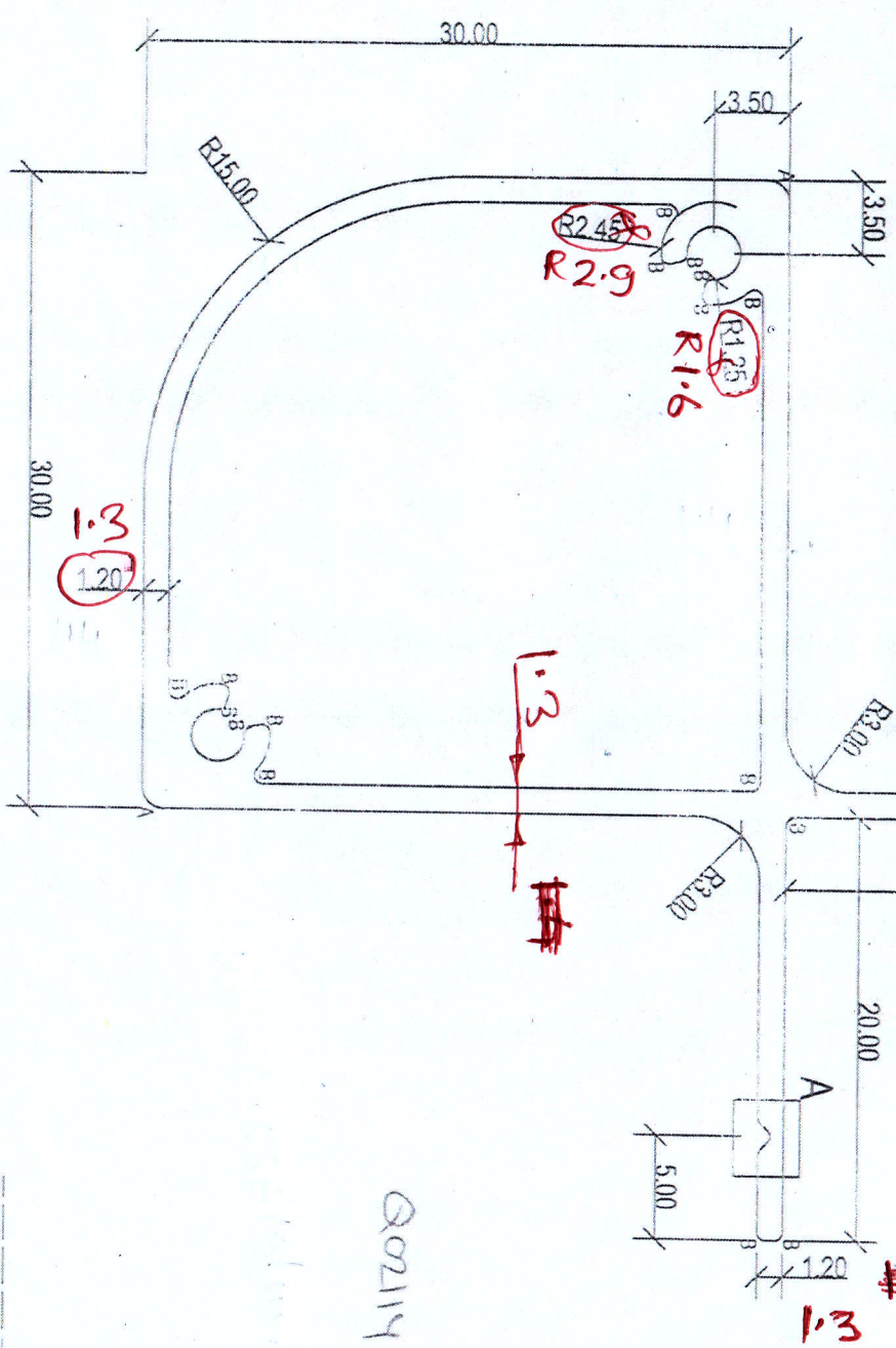
DETAIL: A
