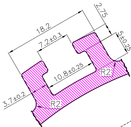
DETAIL-A SCALE 2:1
