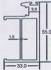
814817 NON STRUCTURE INTERLOCK
