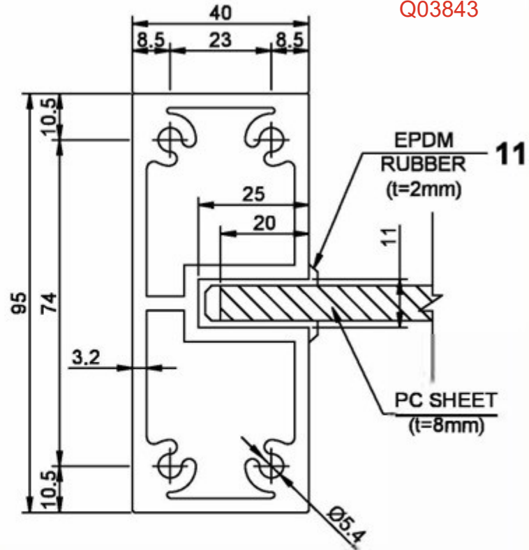
DETAIL - E (SCALE N.T.S.) ALUMINIUM SECTION (SINGLE EXTRUDE)
