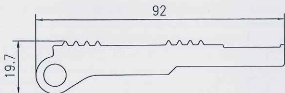
型材轮廓图 1:1
