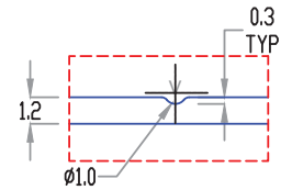
V-GROOVE SCALE 4 : 1
