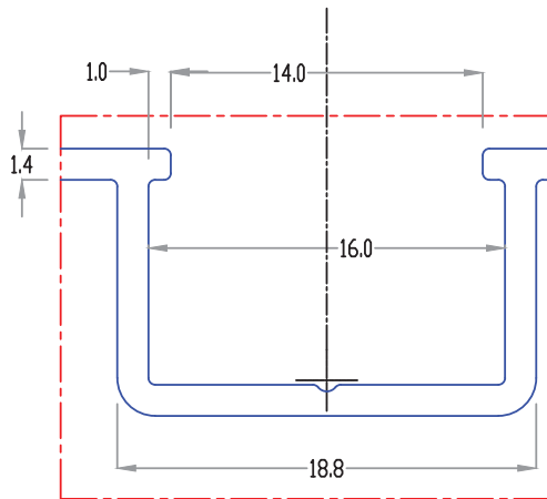
DETAIL-B SCALE 4 : 1
