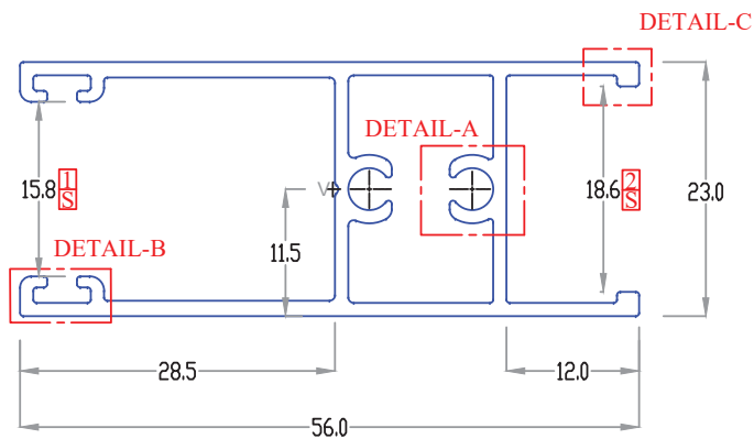
SCALE 2 : 1
