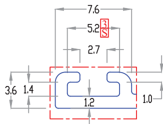
DETAIL-B SCALE 4 : 1
