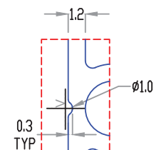
V-GROOVE SCALE 4 : 1
