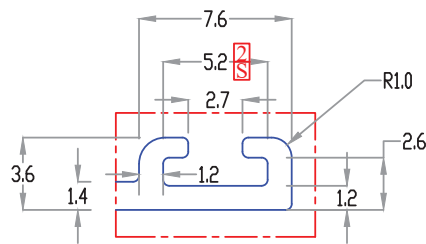
DETAIL-C SCALE 4 : 1
