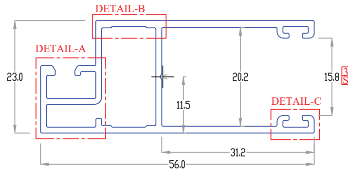
SCALE 2 : 1
