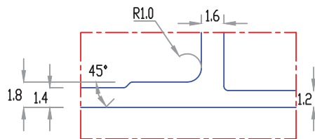
DETAIL-C SCALE 4 : 1
