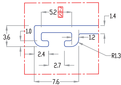
DETAIL-B SCALE 4 : 1
