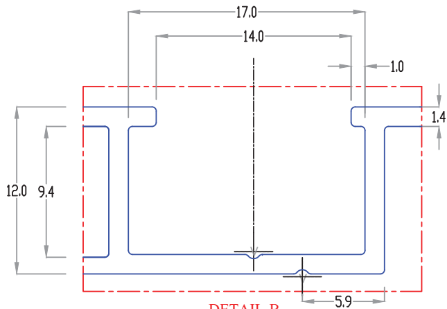
DETAIL-B SCALE 4 : 1
