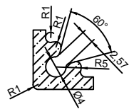
DETAIL VIEW-A SCALE : 2:1
