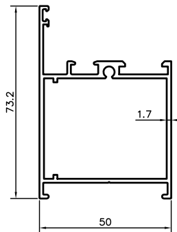
DOOR INSIDE OPEN SASH
