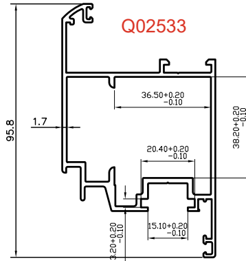
DOOR INSIDE OPEN SASH
