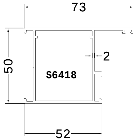
DOOR OUTER
