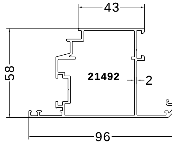
DOOR SASH
