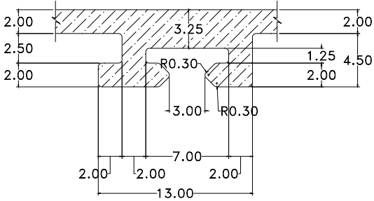
DETAIL-A (SCALE 1:1)
