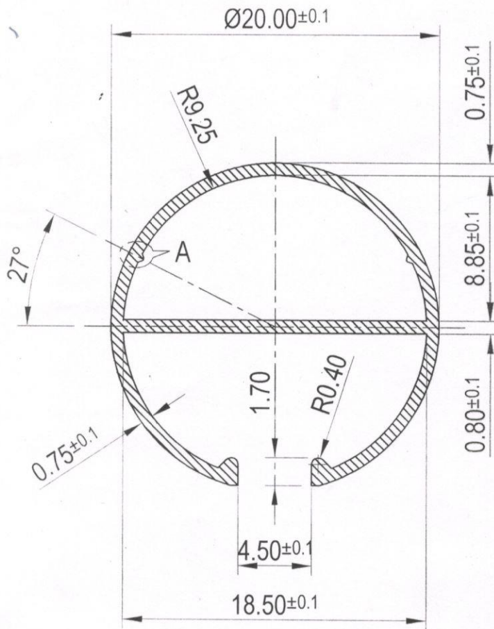
ELAVATION Actual sec. size
