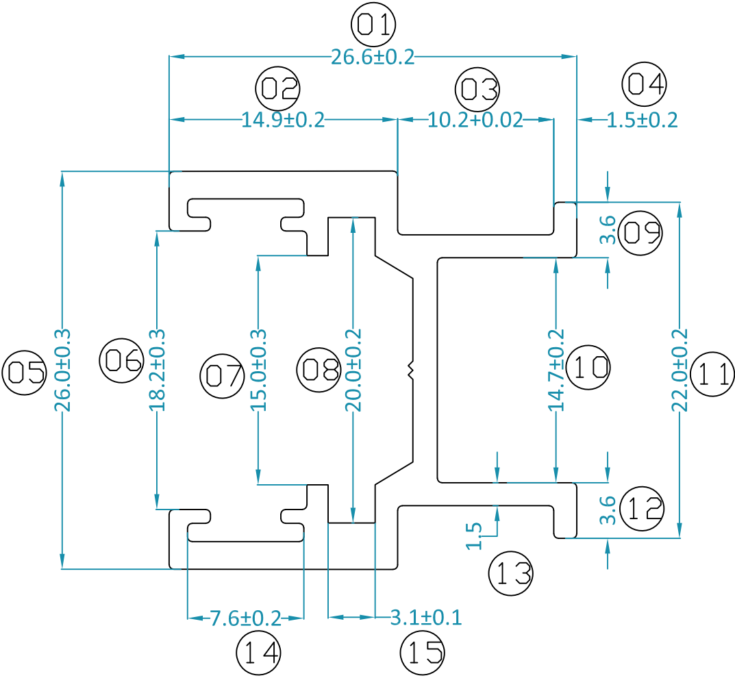
SCALE-3:1
