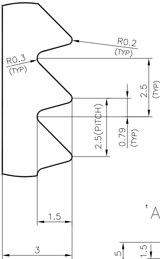
DETAILS 'B' 10:1
