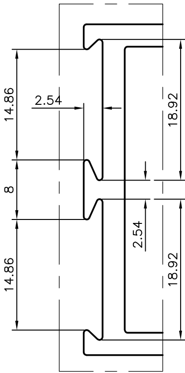
DETAIL-A SCALE: -2:1
