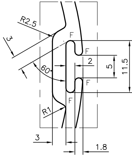
DETAIL-B SCALE: -2:1
