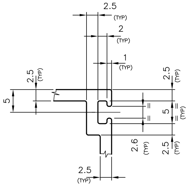
DETAILS A 2:1
