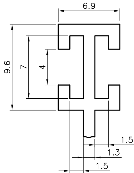
DETAIL-B
