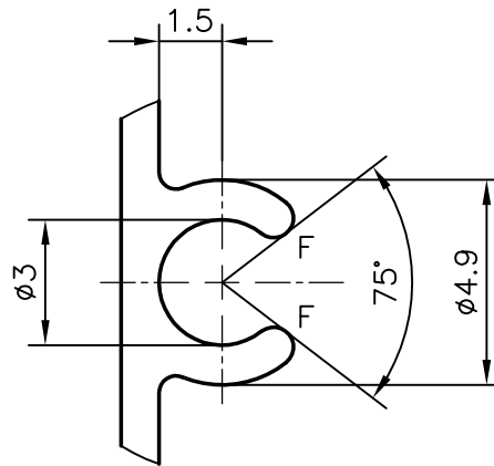
A (5:1) (TYP.)
