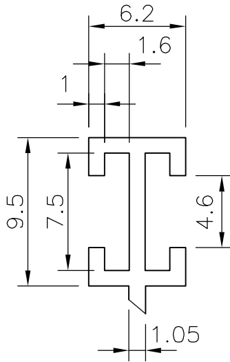
DETAIL 'B' (3:1)
