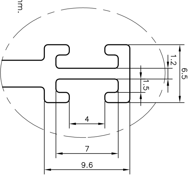
DETAIL-B SCALE:-4:1
