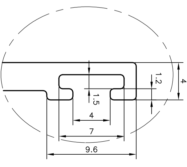
DETAIL-A SCALE:-4:1
