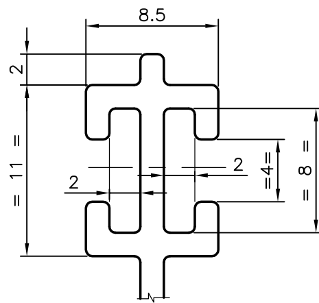
DETAIL-B SCALE:-3:1
