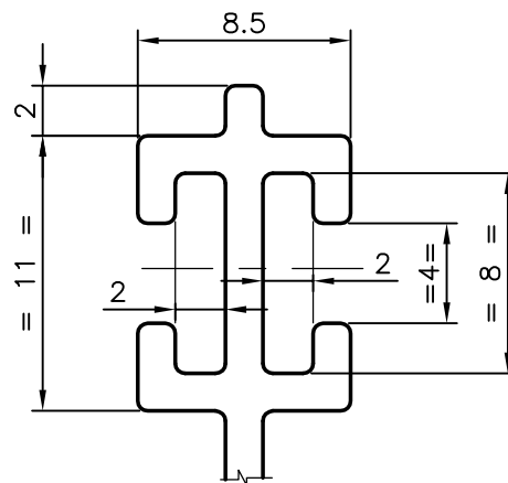
DETAIL-B SCALE:-3:1
