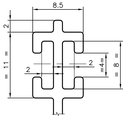
DETAIL-B SCALE:-3:1
