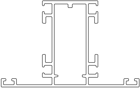
SCALE 1:1
