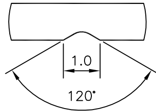
'V' GROOVE DETAIL (10:1)
