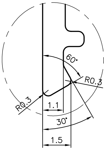
DETAIL-A SCALE: -8:1
