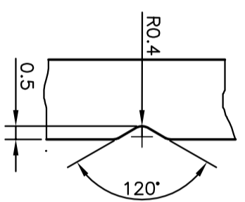
DETAIL 'B' SCALE 5:1
