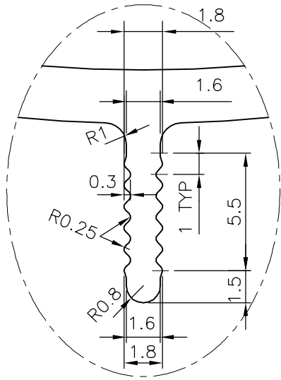
DETAIL-A SCALE: -4:1
