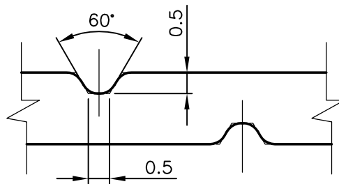
DETAIL-A SCALE:-8:1
