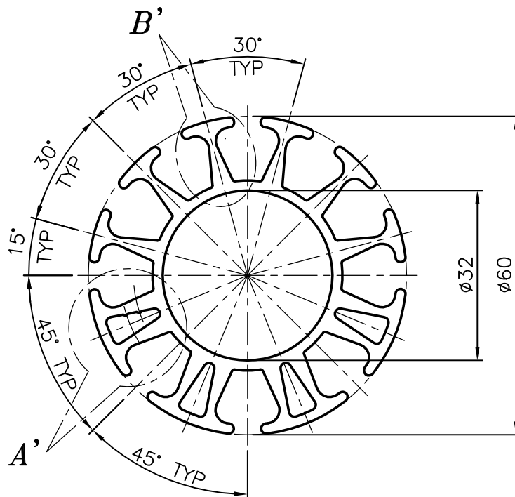
DETAIL-A SCALE:3:1
