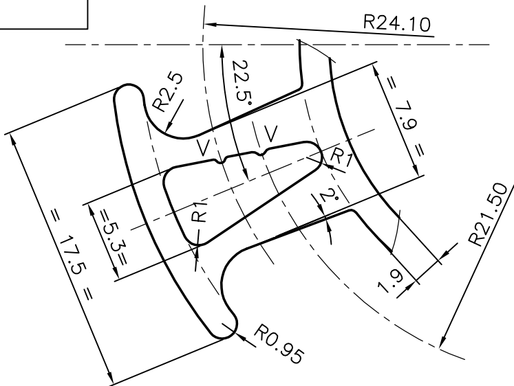
DETAIL-A SCALE:3:1
