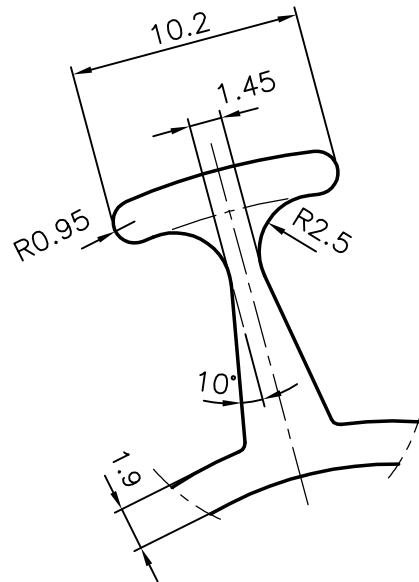
DETAIL-B SCALE:3:1
