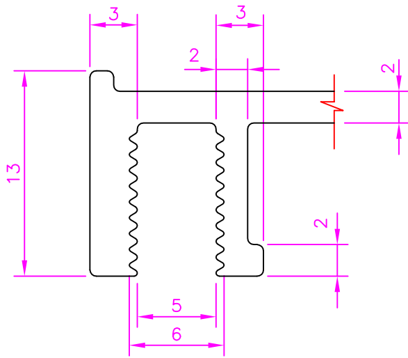
DETAIL-B SCALE:-3:1
