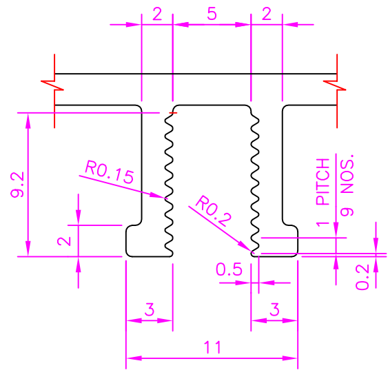
DETAIL-A SCALE:-3:1
