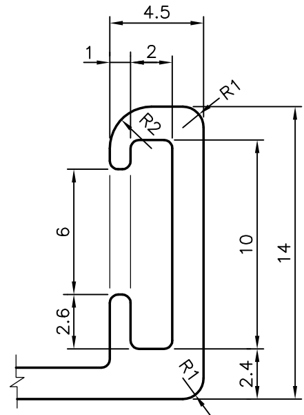
DETAIL-B
