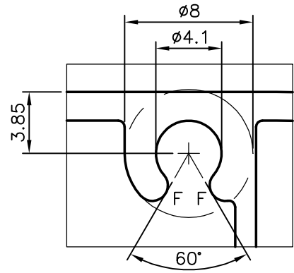
DETAIL-A SCALE: - 3:1
