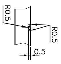
VEE GROOVE DETAIL SCALE 2:1
